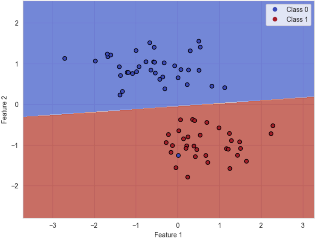
Hard Margin SVM (C=100) <PES2UG23CS333>
